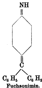
Fuchsonimin.
